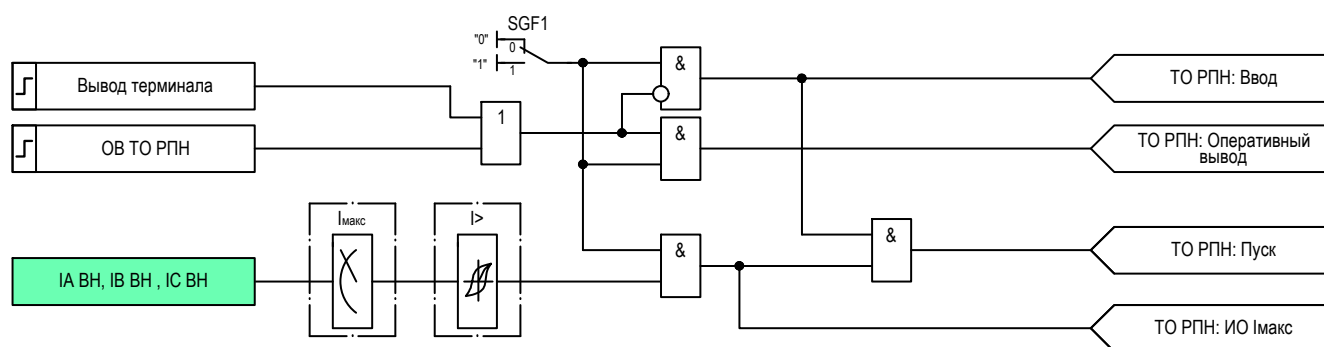
Рисунок 2.17 – Функциональная схема логики ТО РПН
