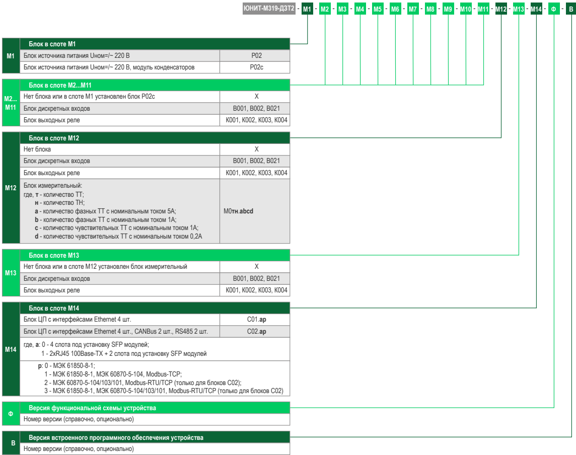
Рисунок Б.2 – Код заказа устройства «ЮНИТ-М319-ДЗТ2»
